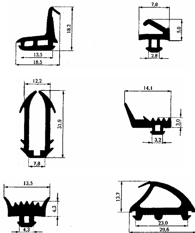
Рисунок А.4 — Уплотнители для оконных и дверных блоков из алюминиевых профилей
