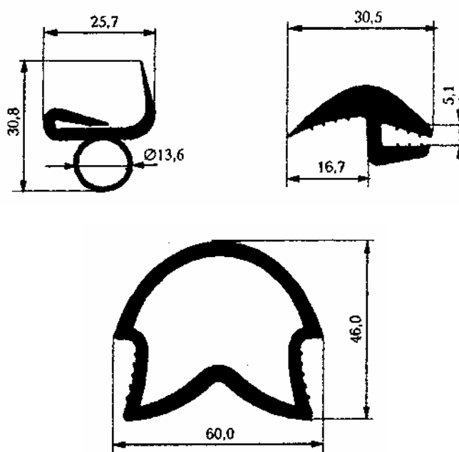
Рисунок А.5 — Уплотнители для теплиц
