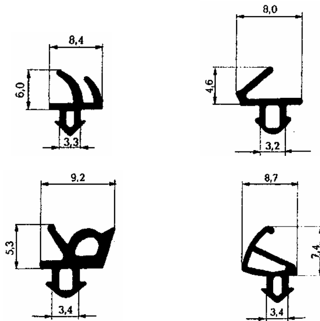
Рисунок А.2 — Уплотнители для поливинилхлоридных оконных и дверных блоков
